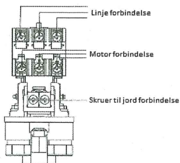
Aluminium flange til tank forbindelse
